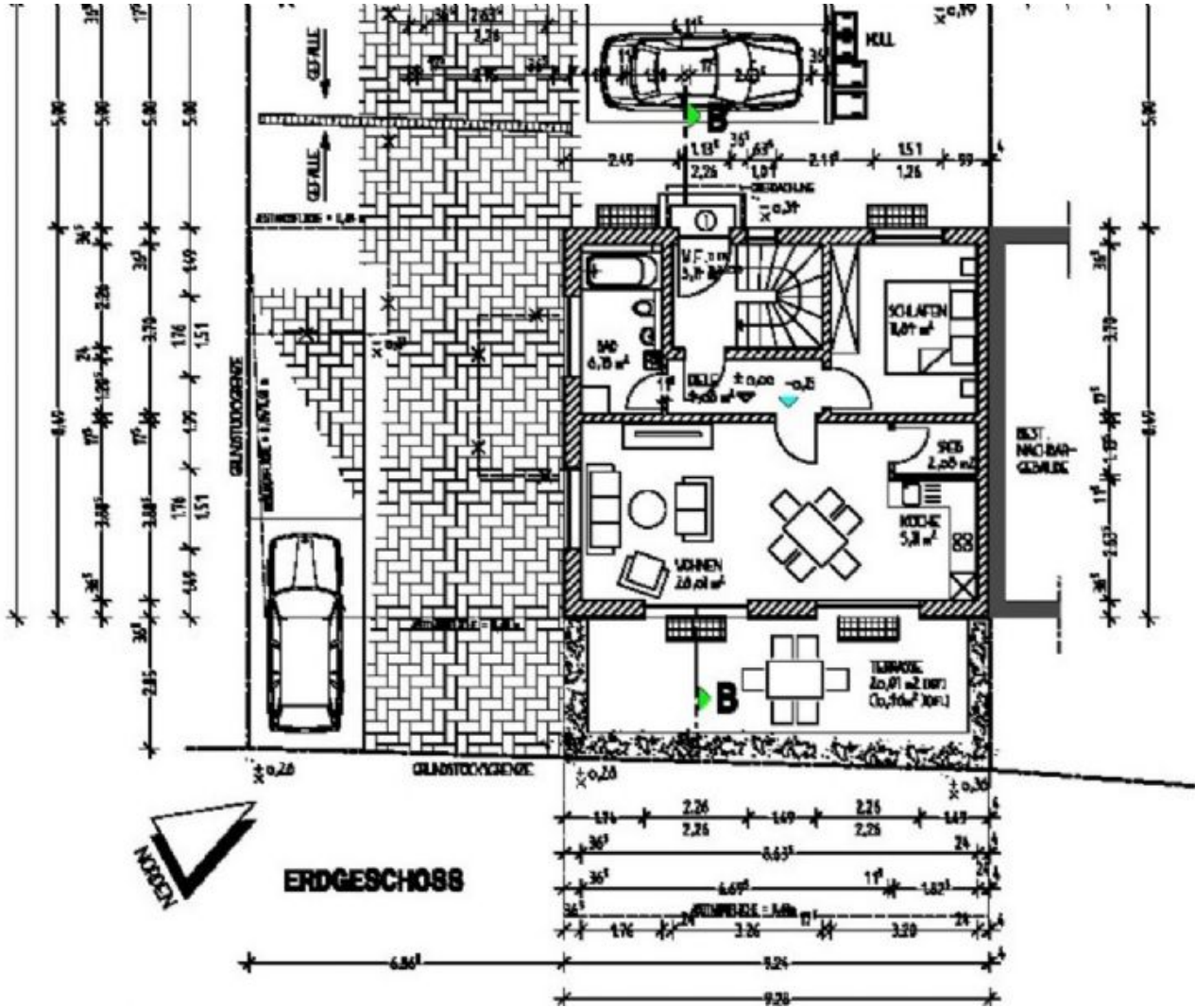
Grundriss Erdgeschoss
