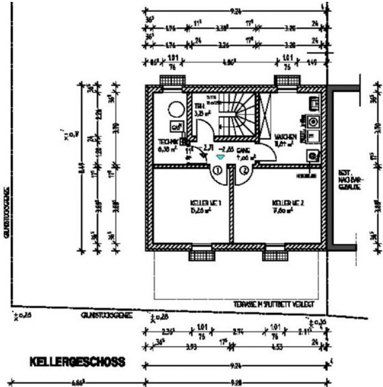
Grundriss Keller
